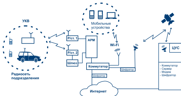
Принципиальная схема МПАКС «Корсар-15»
