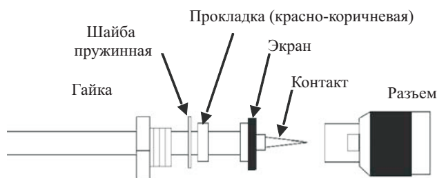
Сборка разъёма
